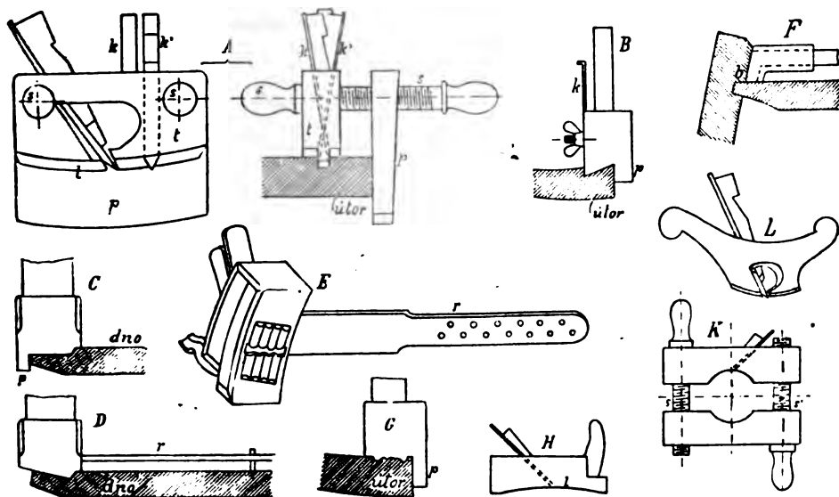
Č. 1729. Hoblíky bednářské a kolářské.
